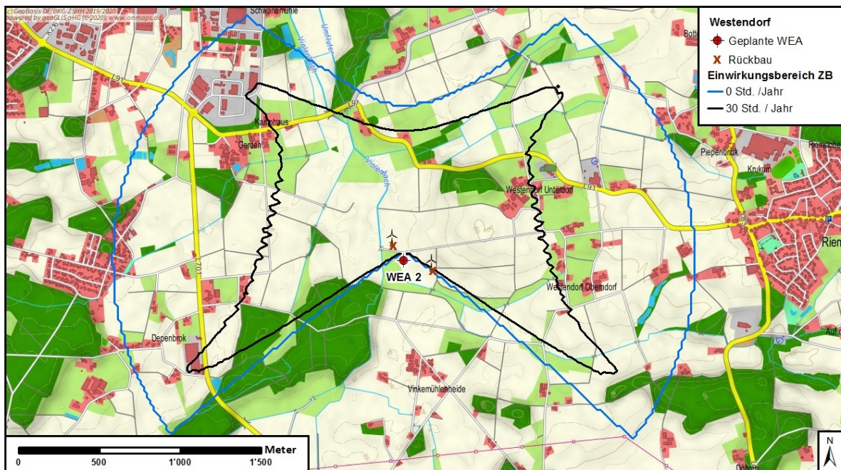
Abbildung 2: Einwirkungsbereich Schattenwurf, Kriterium Stunden pro Jahr
