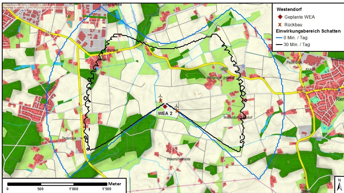
Abbildung 3: Einwirkungsbereich Schattenwurf, Kriterium Minuten pro Tag
